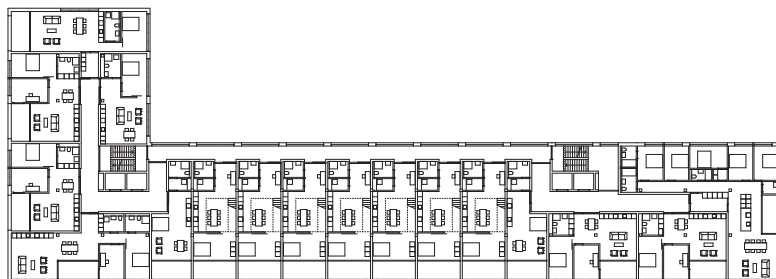
Grundriss neu, Mst. 1:1000.
